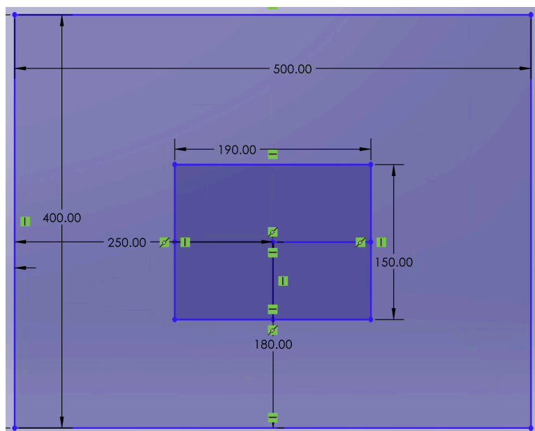
Rectángulo de 500 mm x 400 mm, con abertura rectangular de 190 mm x 150 mm. La abertura está centrada a 250 mm en X y 180 mm en Y desde la esquina inferior izquierda del panel.
